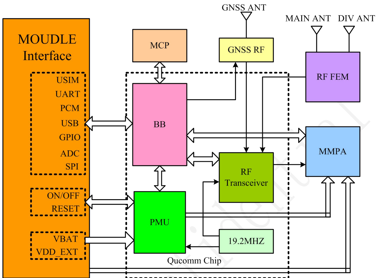
图2-1 CLM920 NC3 LCC模块功能框图
