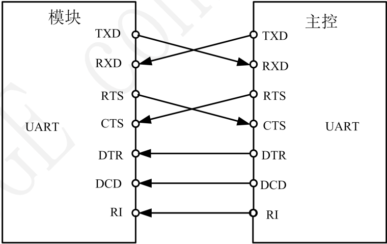
图 3-12 全功能串口设计图
