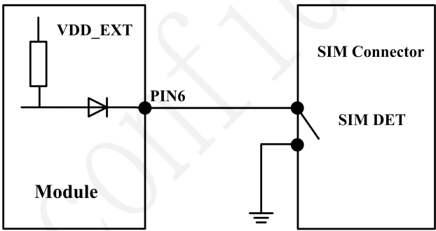
图 3-17 USIM 卡热插拔检测
