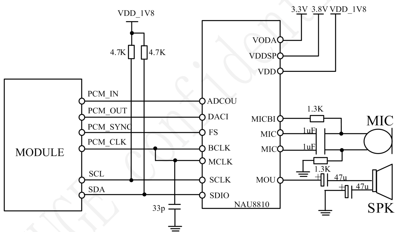
图3- 21 PCM转模拟语音图
