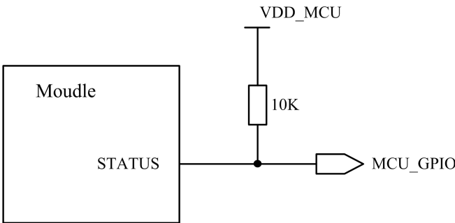
图3-19 STATUS管脚参考电路
