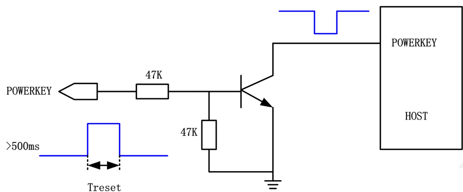
图 3-8 开机参考电路
