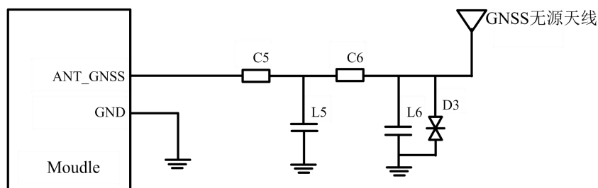
图3-27 GNSS无源天线参考电路
