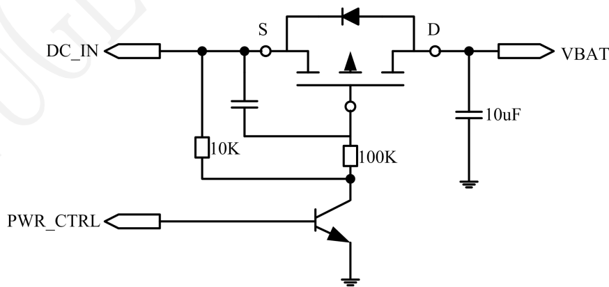
图 3-6 PMOS 管控制电源开关参考电路
