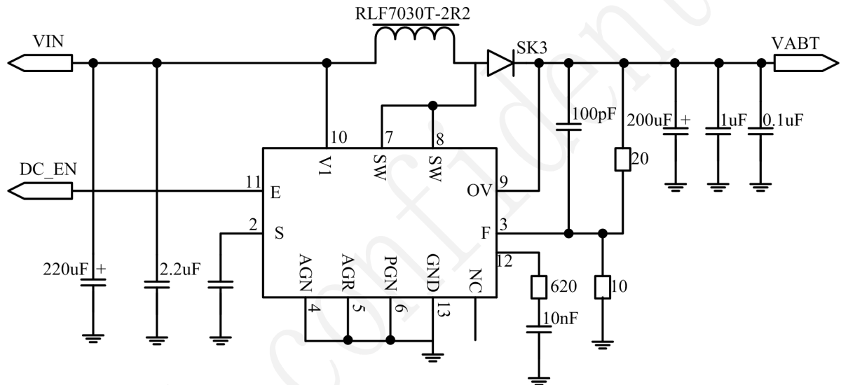
图 3-5 DC 开关电源参考电路
