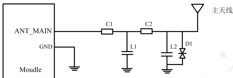
图 3-25 主集天线匹配电路
