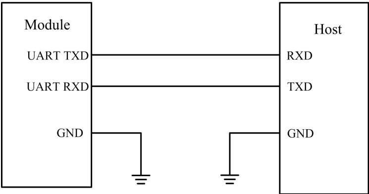
图 3-13 UART 串口设计图
