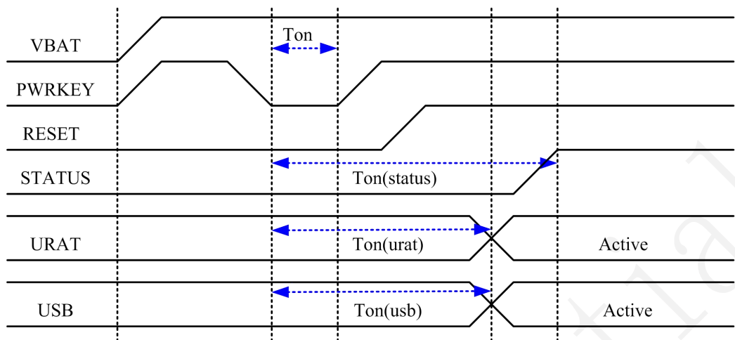
图 3-7 开机时序图
