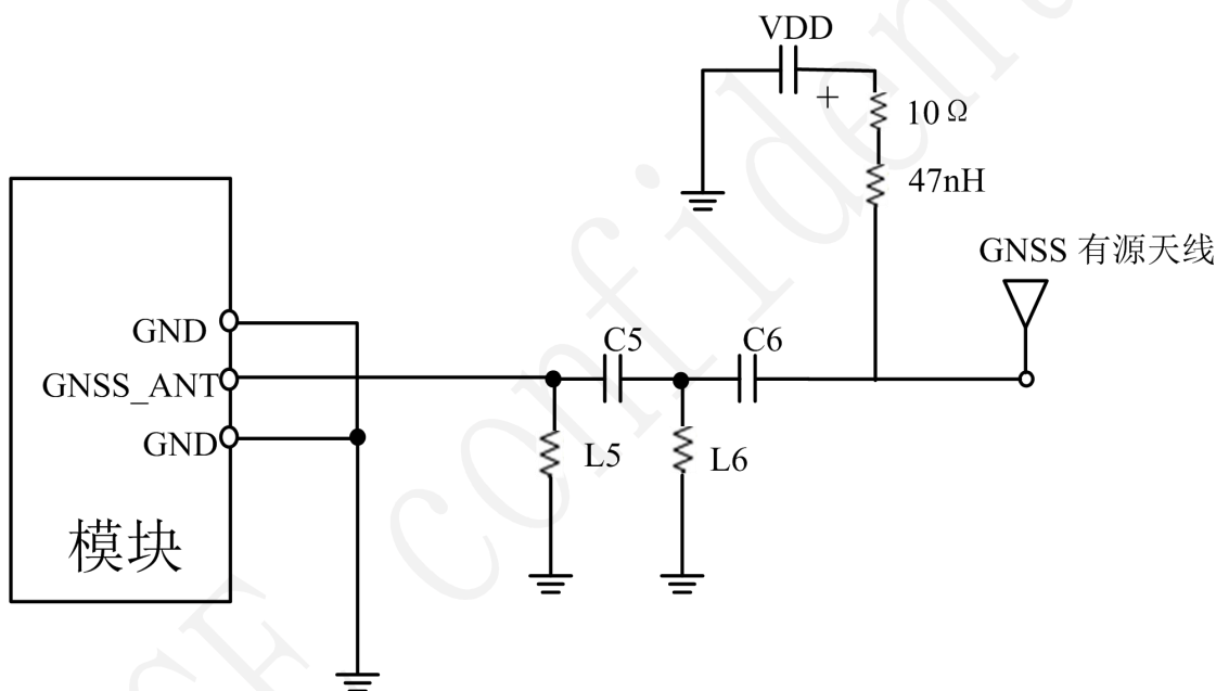
图3-28 GNSS有源天线参考电路
