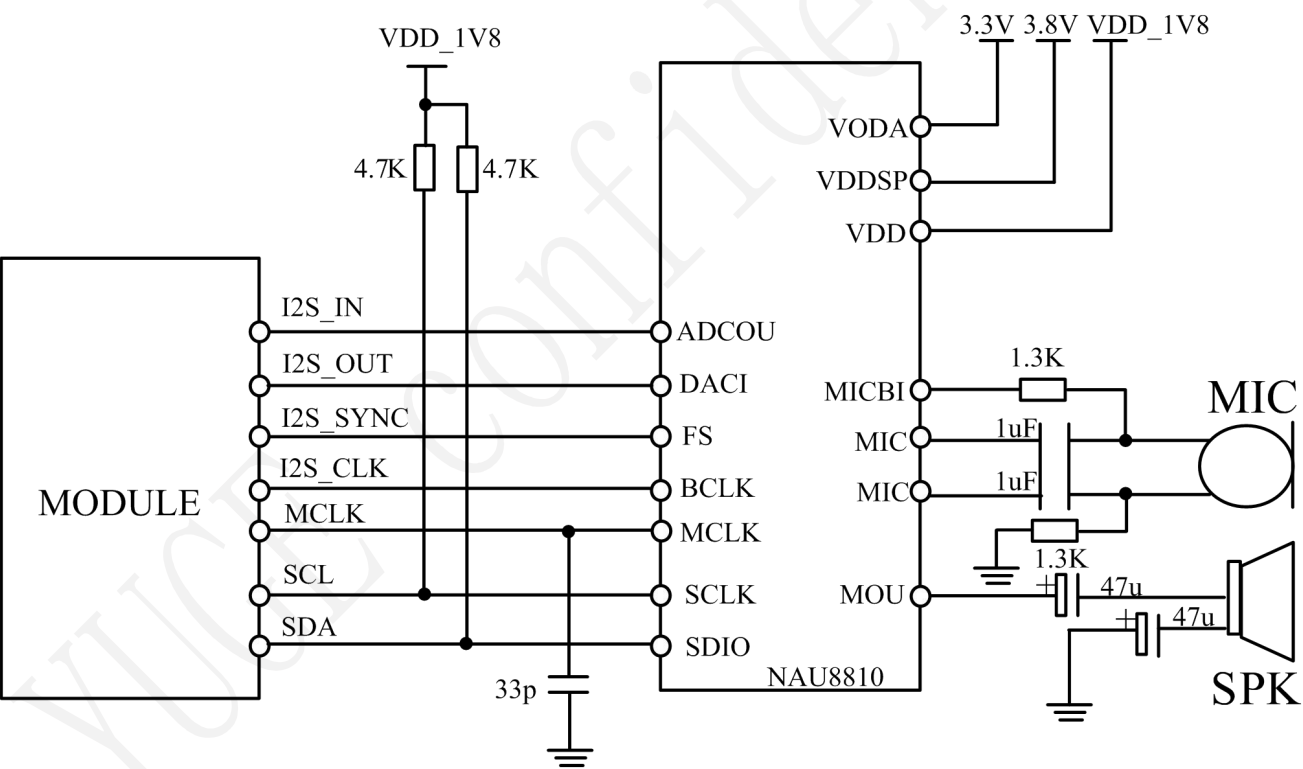
图3-24 I2S转模拟语音图
