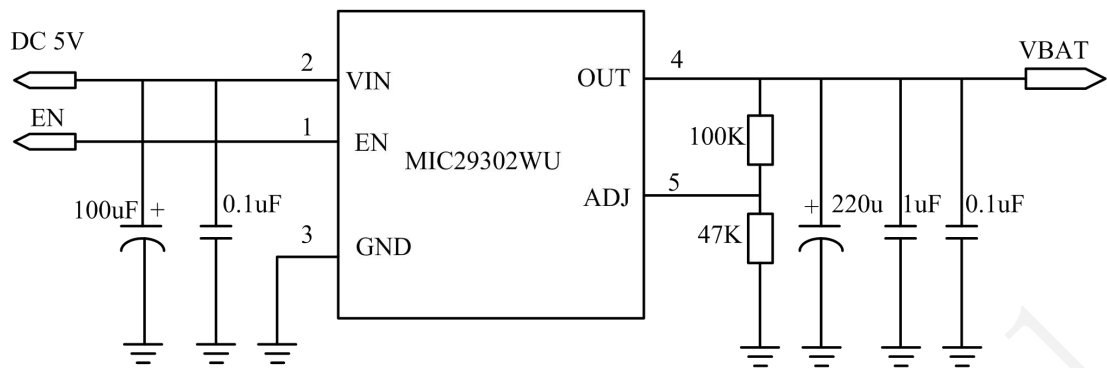
图 3-4 LDO 线性电源参考电路
