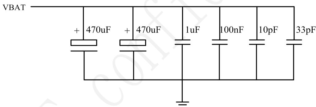
图 3-3 VBAT 供电电源
