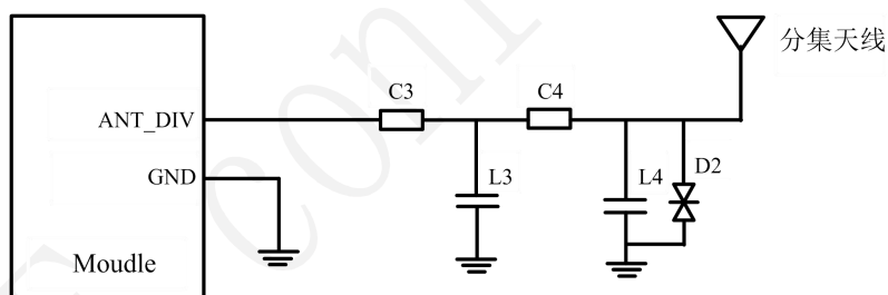
图 3-26 分集天线匹配电路
