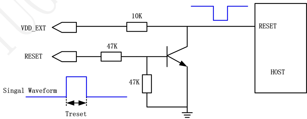
图3-9 复位参考电路
