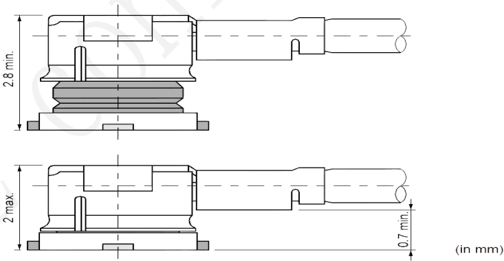
图 3-34 匹配的同轴射频线尺寸
