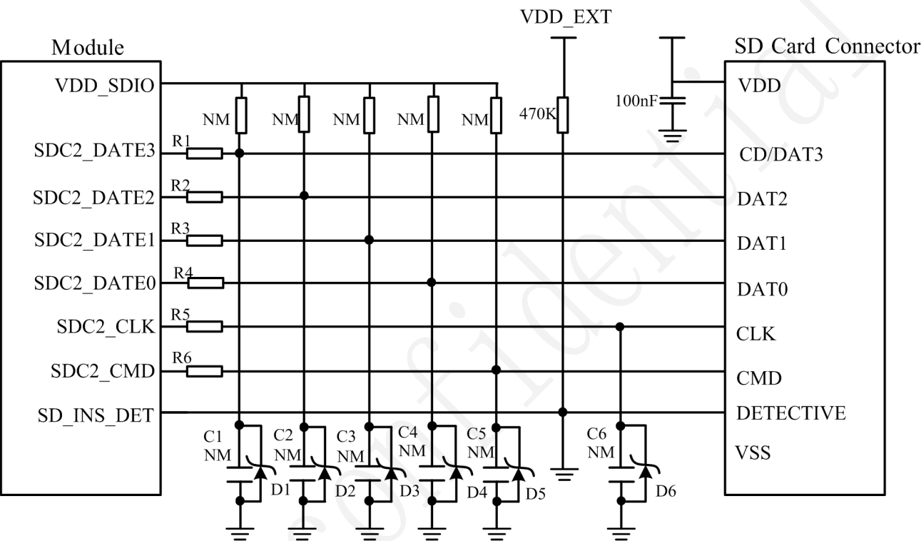
图3-23 SD卡接口参考电路图
