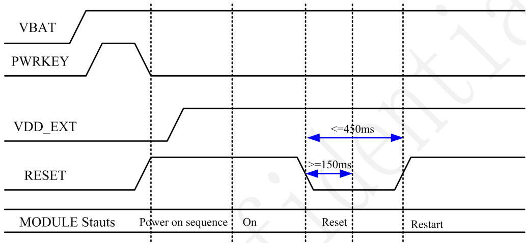
图 3-10 复位时序图
