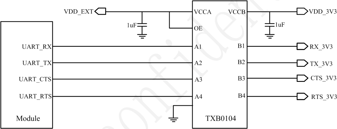
图 3-14 电平转换芯片电路
