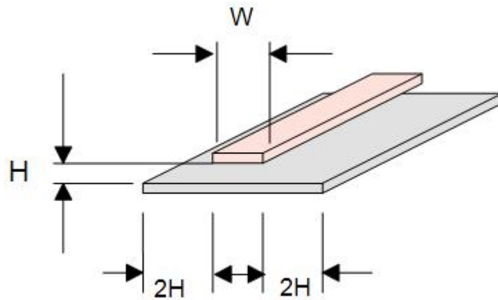
图 3-29 两层 PCB 板微带线的完整结构
