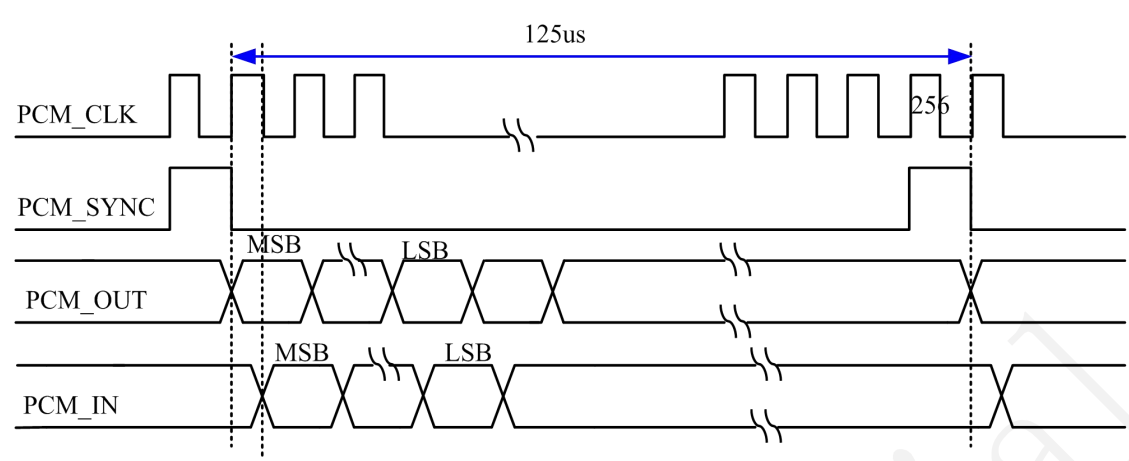
图 3-20 PCM 短帧模式时序图
